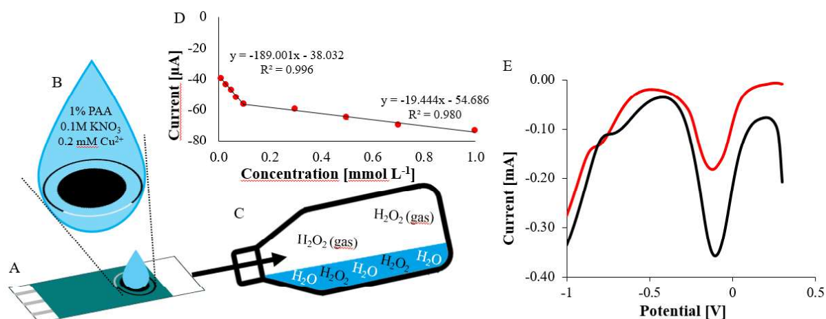
Schemat 2. Schemat układu pomiarowego do detekcji nadtlenu wodoru w fazie gazowej. (A) Elektroda sitodrukowana zawierająca trzy elektrody: węglową elektrodę roboczą, srebrną elektrodę quasi-odniesienia oraz węglową elektrodę pomocniczą, na powierzchnię których naniesiono 50 \mu\text{L} elektrolitu podstawowego zawierającego 1% PAA w 0.1 M \text{KNO}_3 oraz 2 \times 10^{-4} \text{ mol L}^{-1} jonów miedzi(II). (B) Powiększony widok obszaru roboczego systemu (naniesiony roztwór pokrywa powierzchnię wszystkich trzech elektrod). (C) Szczelnie zamknięta szklana komora zawierająca 50 mL wodnego roztworu nadtlenu wodoru o określonym stężeniu. Po 3 godzinach stabilizacji elektroda z naniesionym roztworem była umieszczana wewnątrz komory. (D) Odpowiedź prądowa w funkcji stężenia nadtlenu wodoru rozpuszczonego w elektrolicie podstawowym ( 1 \times 10^{-5} - 1 \times
